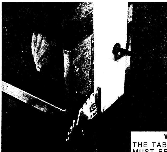
END MORTISING
